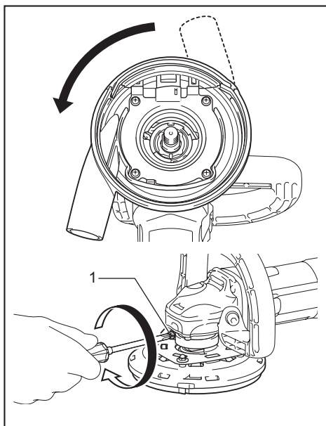
► 1. Tornillo
