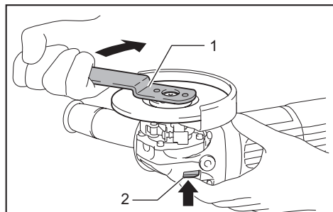
► 1. Clé à contre-écrou 2. Blocage de l'arbre
