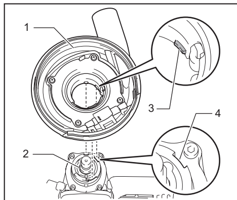
► 1. Protector recolector de polvo de la rueda 2. Caja de cojinetes 3. Protuberancia 4. Muesca
