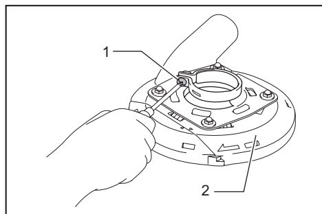
► 1. Tornillo 2. Protector recolector de polvo de la rueda
